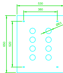
Detalle apoyo Gabinete
