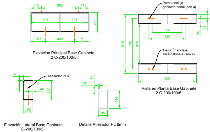
Detalle Perfil Canal L: 0.6 m
