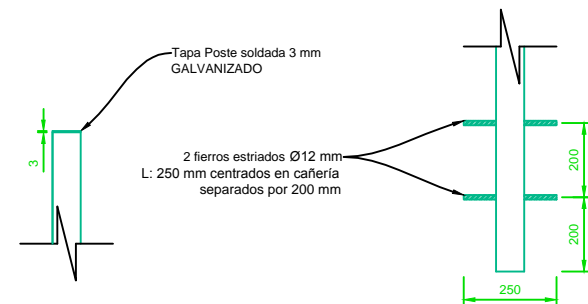
Detalle Poste Antena Satelital L: 2.5 m
